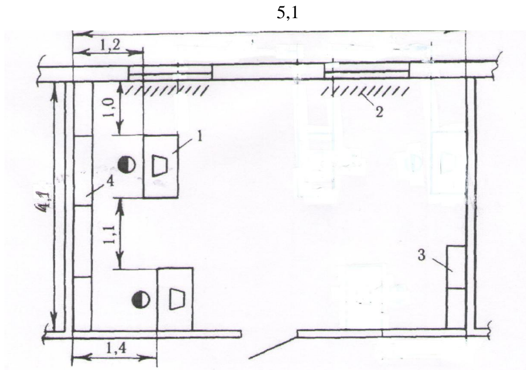
Рис. 4.1. План приміщення з комп'ютеризованими робочими місцями:
