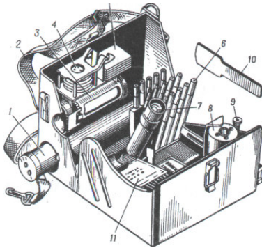
Рис. 5.9 Військовий прилад хімічної розвідки (ВПХР)
