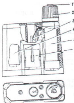
Рис. 5.7 Зарядний пристрій ЗД-6 до комплекту ІД-1
