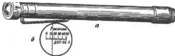
Рис. 5.4. Дозиметр ДКП-50А: a - загальний вигляд; б - шкала
