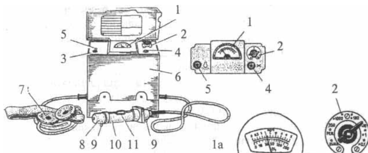
Рис. 5.1. Прилад ДП-5В
