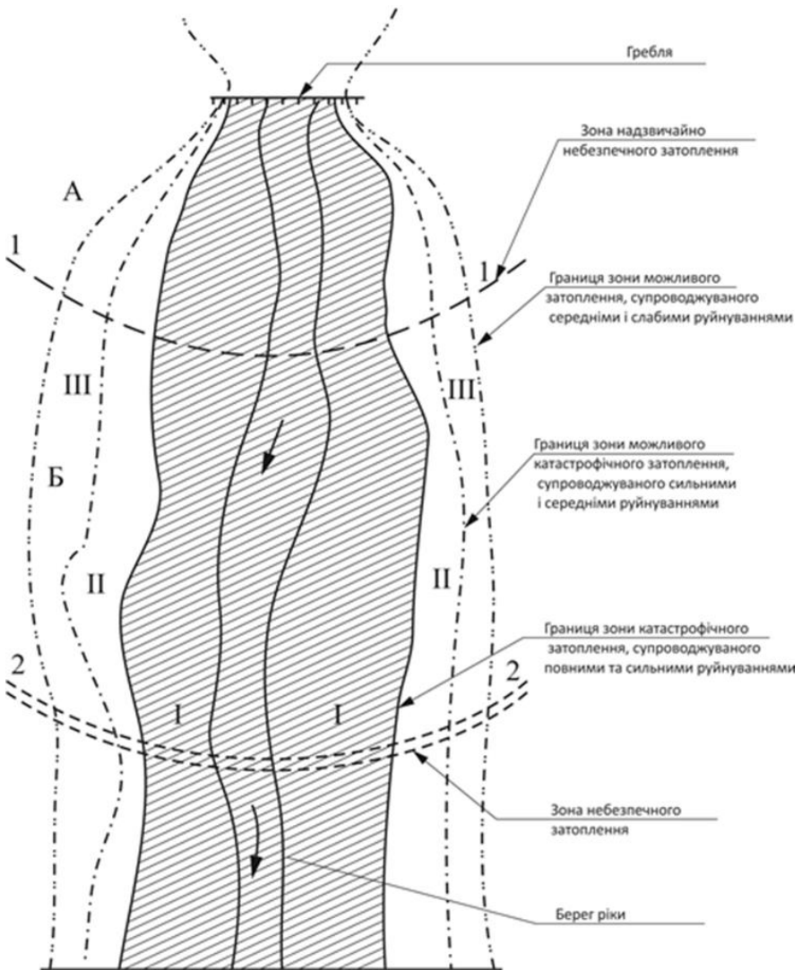
Рисунок 2.2 – Схема зони можливого затоплення при прориві або руйнуванні греблі гідровузла
