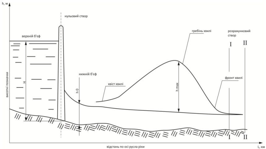
Рисунок 2.1 – Схематичний поздовжній розріз хвилі прориву
